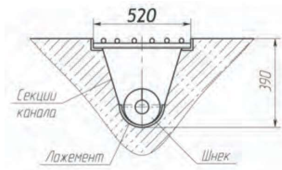
Сечение продольного канала
